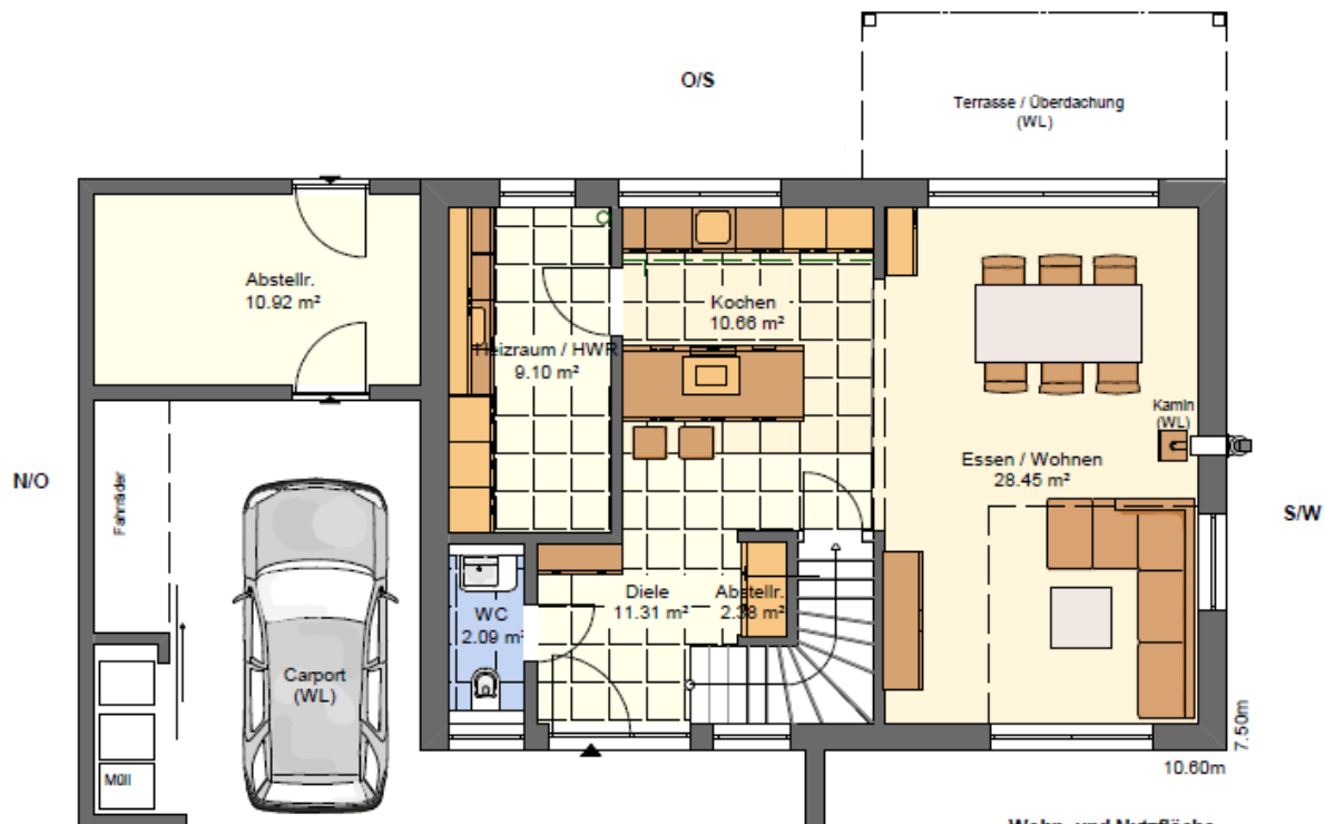
Grundriss Erdgeschoss
