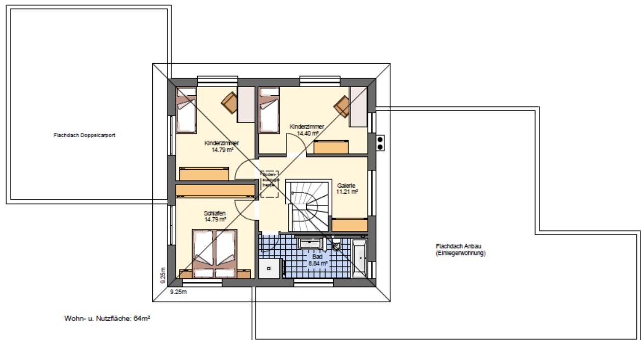
Grundriss Obergeschoss
